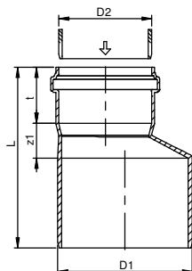
PPKGR – redukce nesouosá dlouhá
