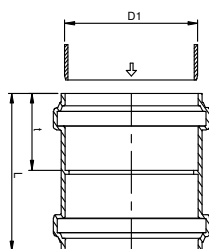
PPKGMM – spojka dvouhrdlá
