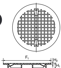
PP poklop A15 – do šachtové roury
