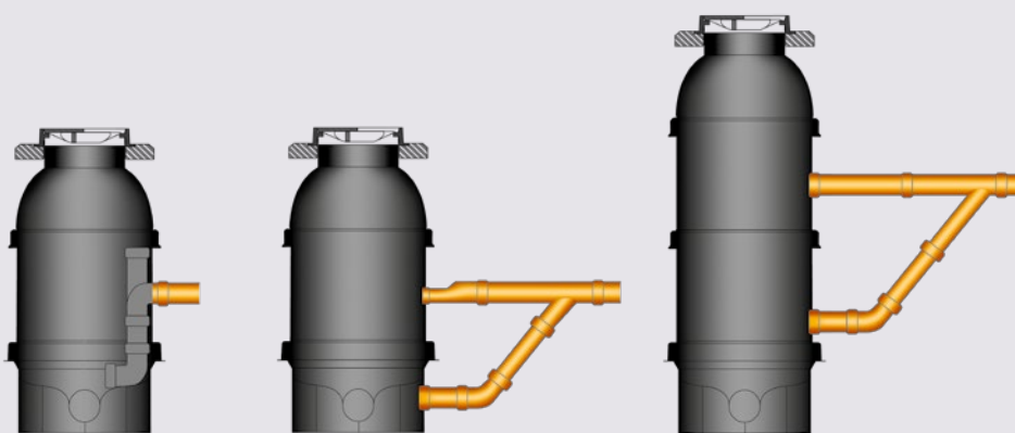
Ukřzkovř řeřenř spadiřřřvř vstupnř řachtŷ
